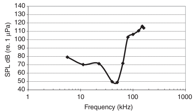
Fig. 7. Audiogram of M. densirostris .
