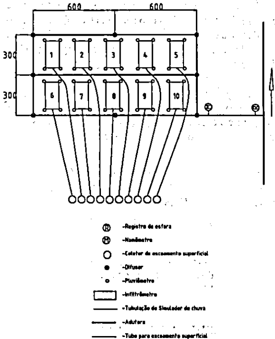
FIG. 1. Esquema experimental utilizado, destacando a posição dos infiltrômetros e coletores de escoamento superficial.
