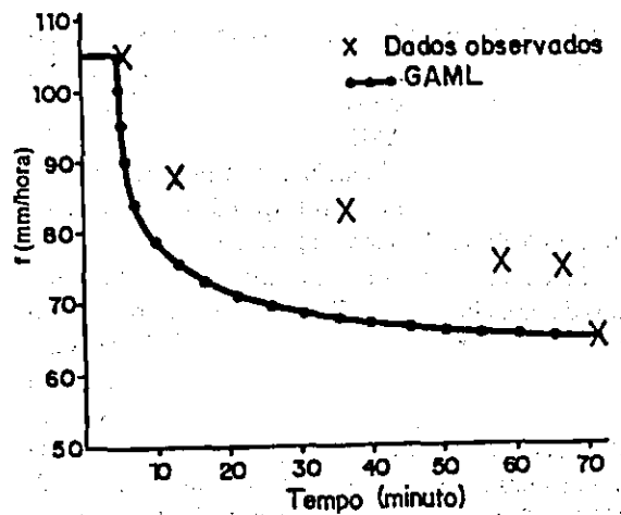
FIG. 4. Valores observados e curva de velocidade de infiltração ( f ) simulada pelo modelo GAML, em um solo provido de cobertura vegetal morta, referentes ao infiltrômetro 10.
