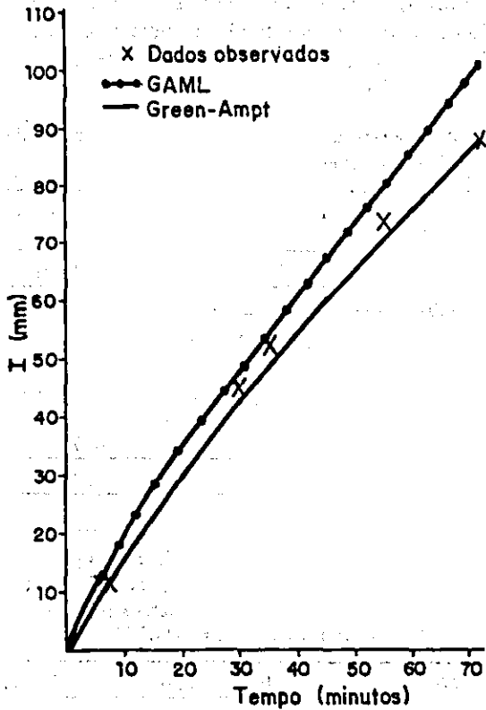
FIG. 3. Valores observados e curvas de infiltração acumulada ( I ) simuladas pelos modelos GAML e Green-Ampt, em um solo desprovido de cobertura vegetal, referentes ao infiltrômetro 2.
