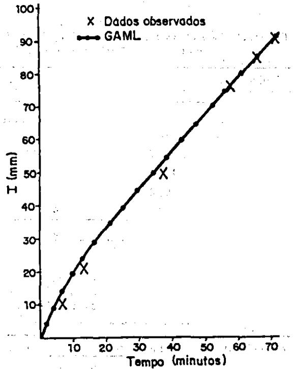
FIG. 5. Valores observados e curva de infiltração acumulada ( I ) simulada pelo modelo GAML, em um solo provido de cobertura vegetal morta, referentes ao infiltrômetro 10.
