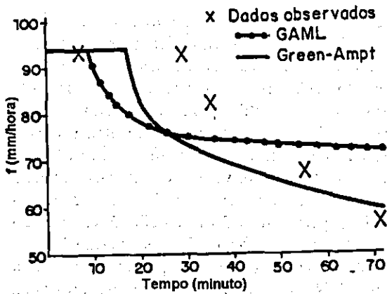
FIG. 2. Valores observados e curvas de velocidade de infiltração ( f ) simuladas pelos modelos GAML e Green-Ampt, em um solo desprovido de cobertura vegetal, referentes ao infiltrômetro 2.
