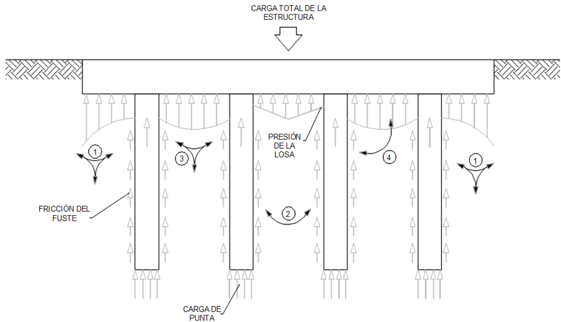
Figura 8. Losas de fundación combinadas con pilotes
