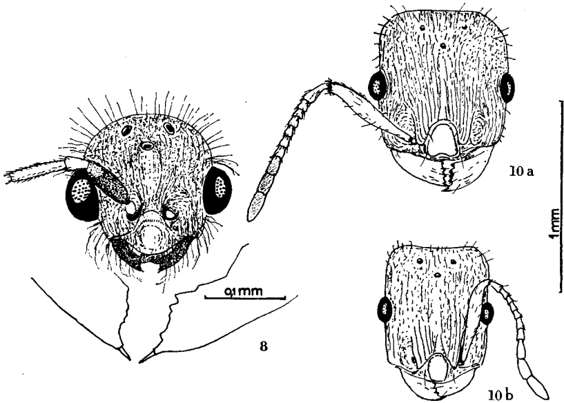
Fig. 8, 10 a und 10 b. Leptothorax , Kopf von vorn. — 8. L. goesswaldi n. sp., ♂, — 10 a. L. goesswaldi n. sp., ♀. — 10 b. L. kutteri BUSCH., ♀.
