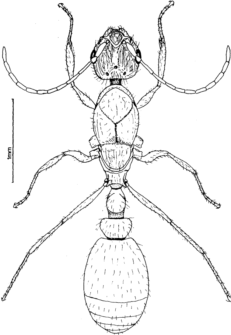
Fig. 15. Leptothorax buschingeri n. sp. ♂ aus dem Laggintal.
