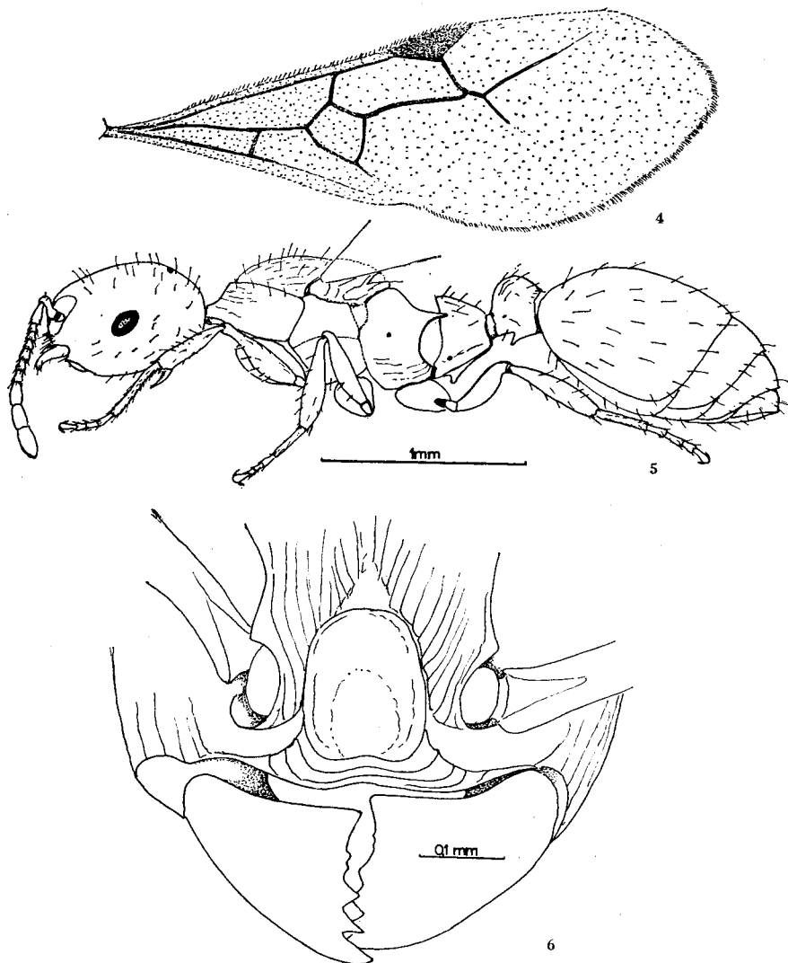
Fig. 4-6. Leptothorax goesswaldi n. sp. ♀.
