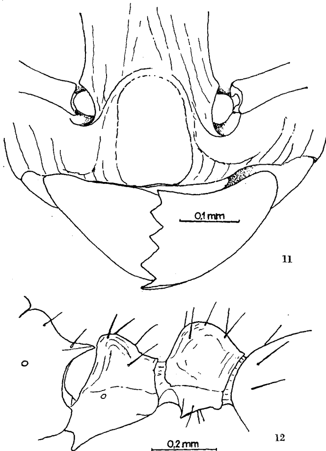
Fig. 11 und 12. Leptothorax kutteri BUSCH., ♀. — 11. Kopfschild und Mandibeln. — 12. Stielchen.
