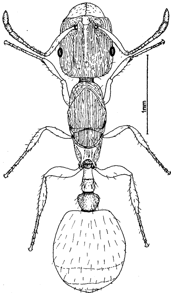
Fig. 3. Leptothorax goesswaldi n. sp. ♀.
