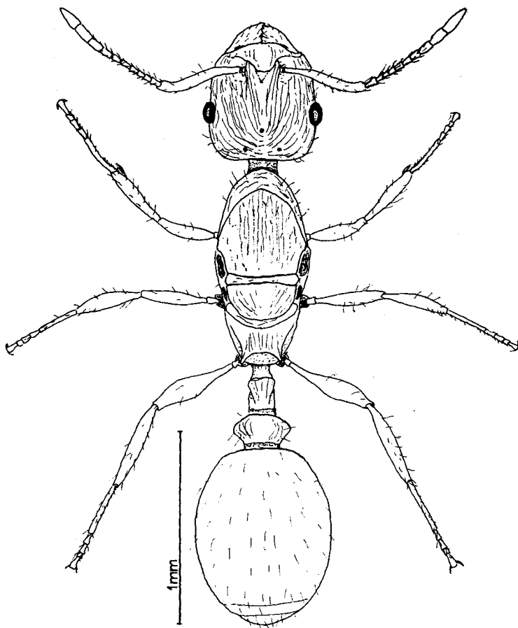
Fig. 9. Leptothorax kutteri BUSCHINGER, ♀.
