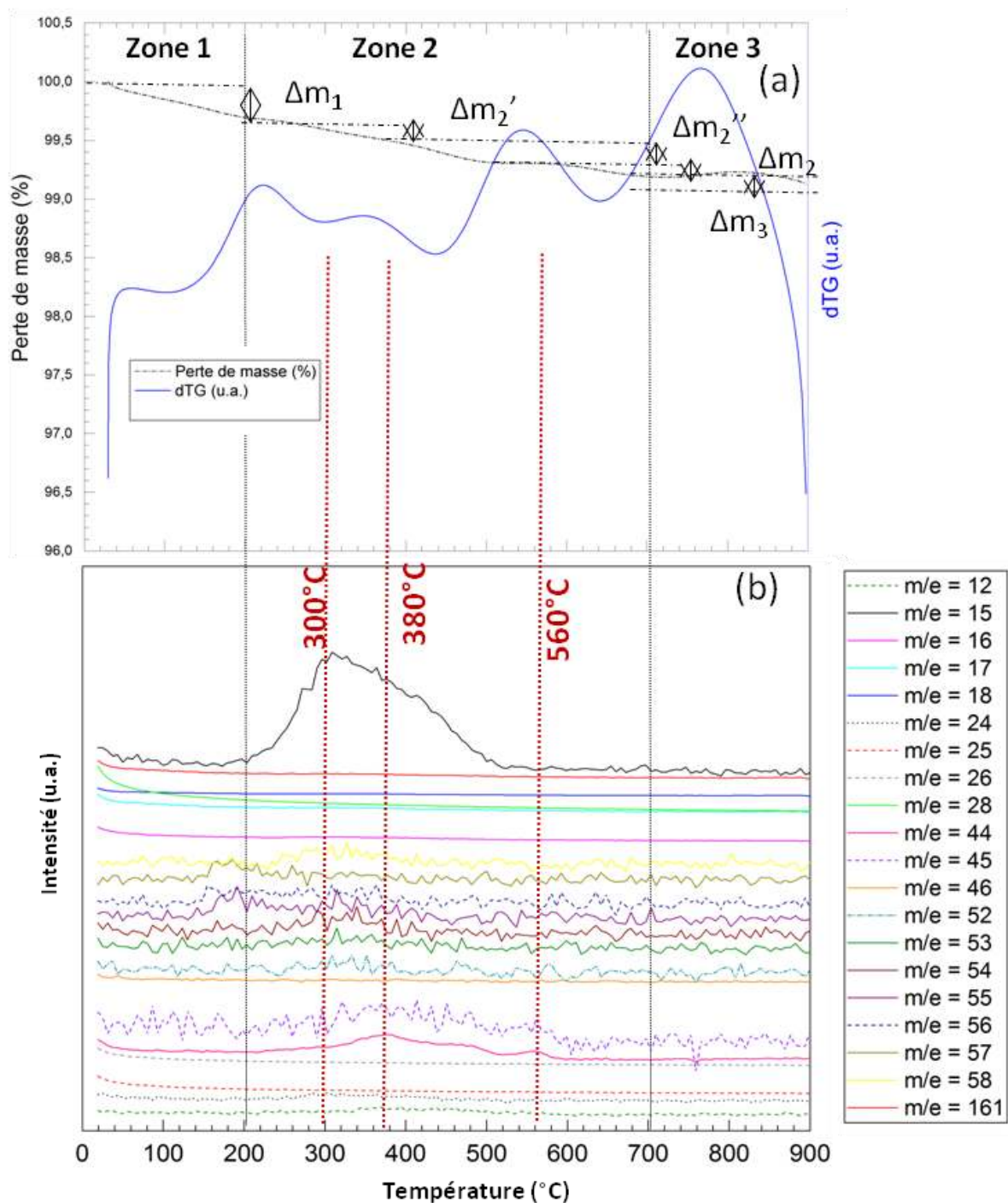
Figure III-15 : (a) Perte de masse (TG), dérivée du signal (dTG) et (b) émissions de masses (SM) des poudres HA-M
