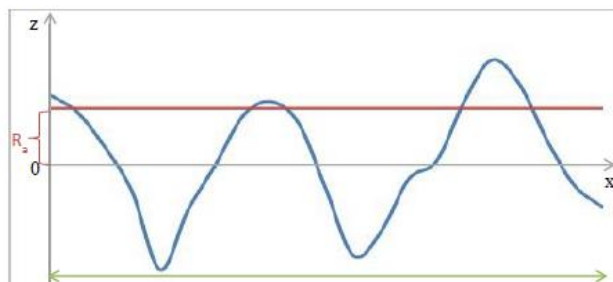
Figure II-2 : Profil linéaire d'une topographie de surface réalisée par AFM permettant le calcul du Ra
