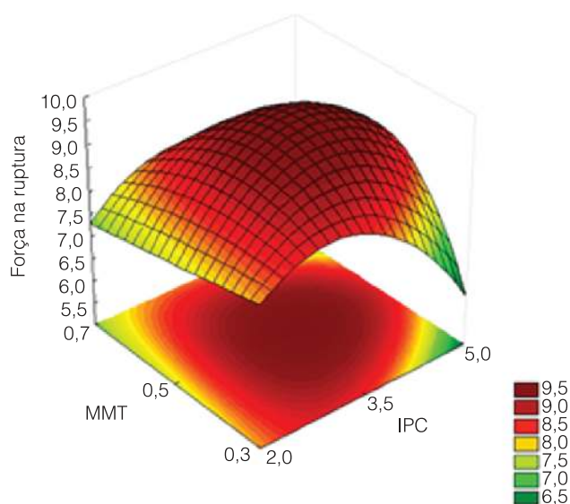
Figura 3. Superfície de resposta da força na ruptura em função das concentrações de MMT (%) e IPC (%) (concentração de glicerol fixa em 30 g.100 g -1 de IPC).
