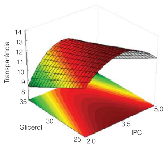
Figura 5. Superfície de resposta da transparência em função das concentrações de glicerol (%) e IPC (%) (concentração de MMT fixa em 0,3%).
