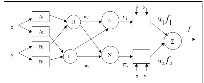
Şekil 1: ANFIS mimarisi.
