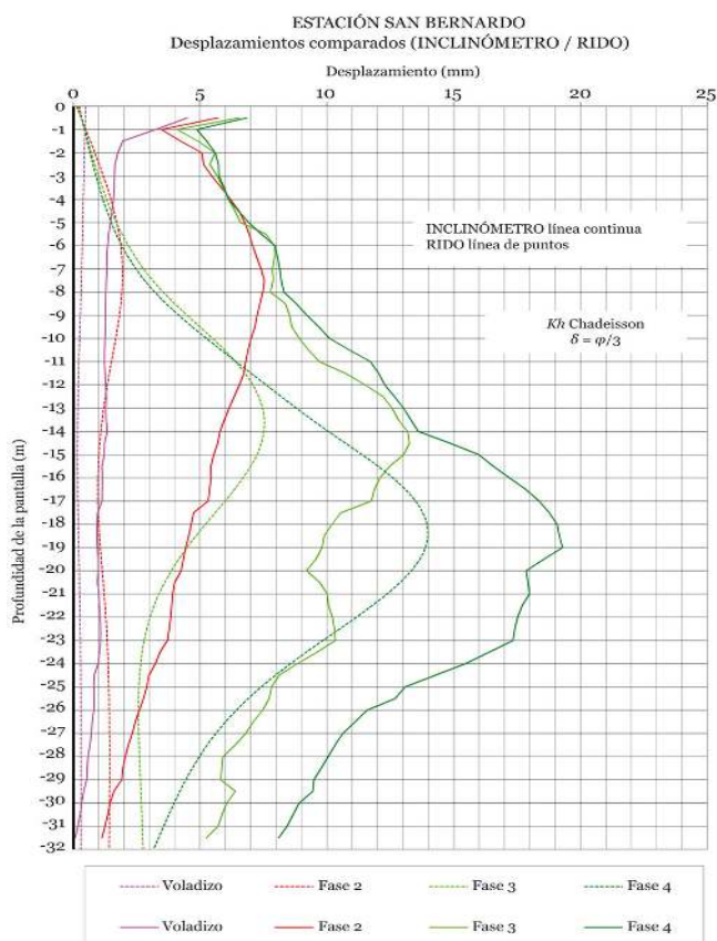
Figura 3. Estación San Bernardo. Desplazamientos comparados Inclinómetro / Rido.
