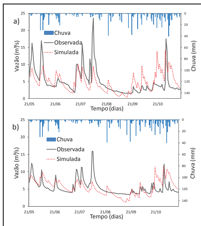
Figure 7 – Método Proxy-catchment. Calibração (a) com os dados da estação Rio Negrinho Montante e validação (b) com os dados do exutório da bacia
