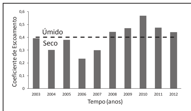
Figura 4 – Coeficiente de escoamento anual usada na divisão dos anos secos e úmidos. A linha tracejada representa a média geral de todos os anos
