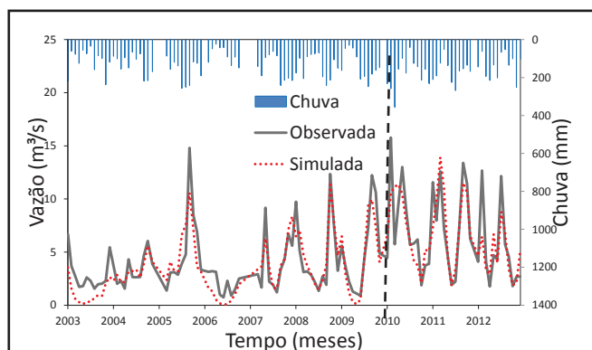
Figura 5 – Processo de calibração e validação mensal. Calibração (2003-2009) e validação (2010-2012)
