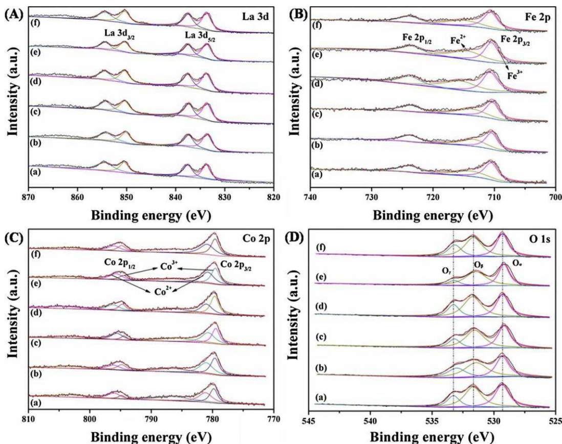
Fig. 5. (A) La 3d, (B) Fe 2p, (C) Co 2p and (D) O 1s XPS spectra of (a) 3DOM LSFCO, (b) 5Co 3 O 4 /3DOM LSFCO, (c) 8Co 3 O 4 /3DOM LSFCO, (d) 10Co 3 O 4 /3DOM LSFCO, (e) 12Co 3 O 4 /3DOM LSFCO, and (f) 16Co 3 O 4 /3DOM LSFCO.
