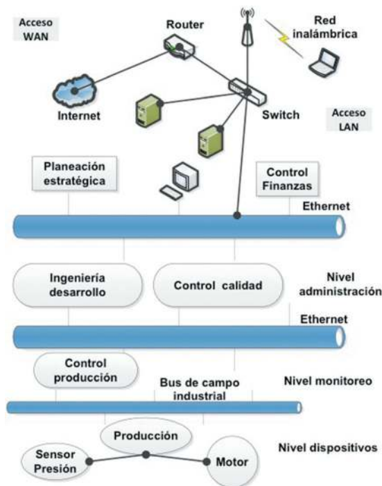
Fig. 3. RED INDUSTRIAL CONFIGURADA CON ETHERNET Y ACCES
