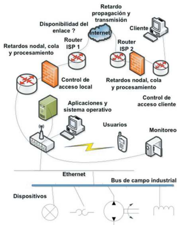
Fig. 4. ELEMENTOS PRESENTES EN UN SISTEMA DE COMUNICACIONES DE MONITOREO VIA WEB
