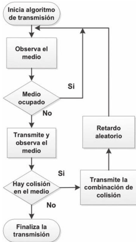
Fig. 1. MODO DE OPERACIÓN DEL ACCESO AL MEDIO CSMA/CD
