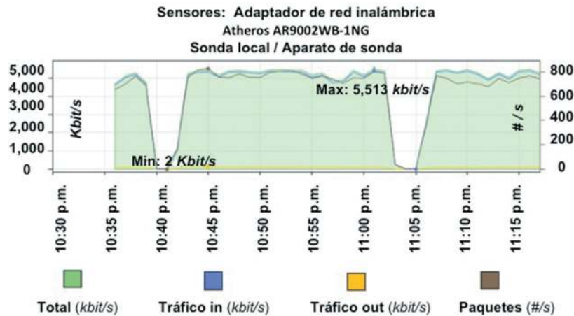
Fig. 2. CANTIDAD DE TRÁFICO E INTERRUPCIÓN DEL FLUJO ANALIZADO CON PRTG
