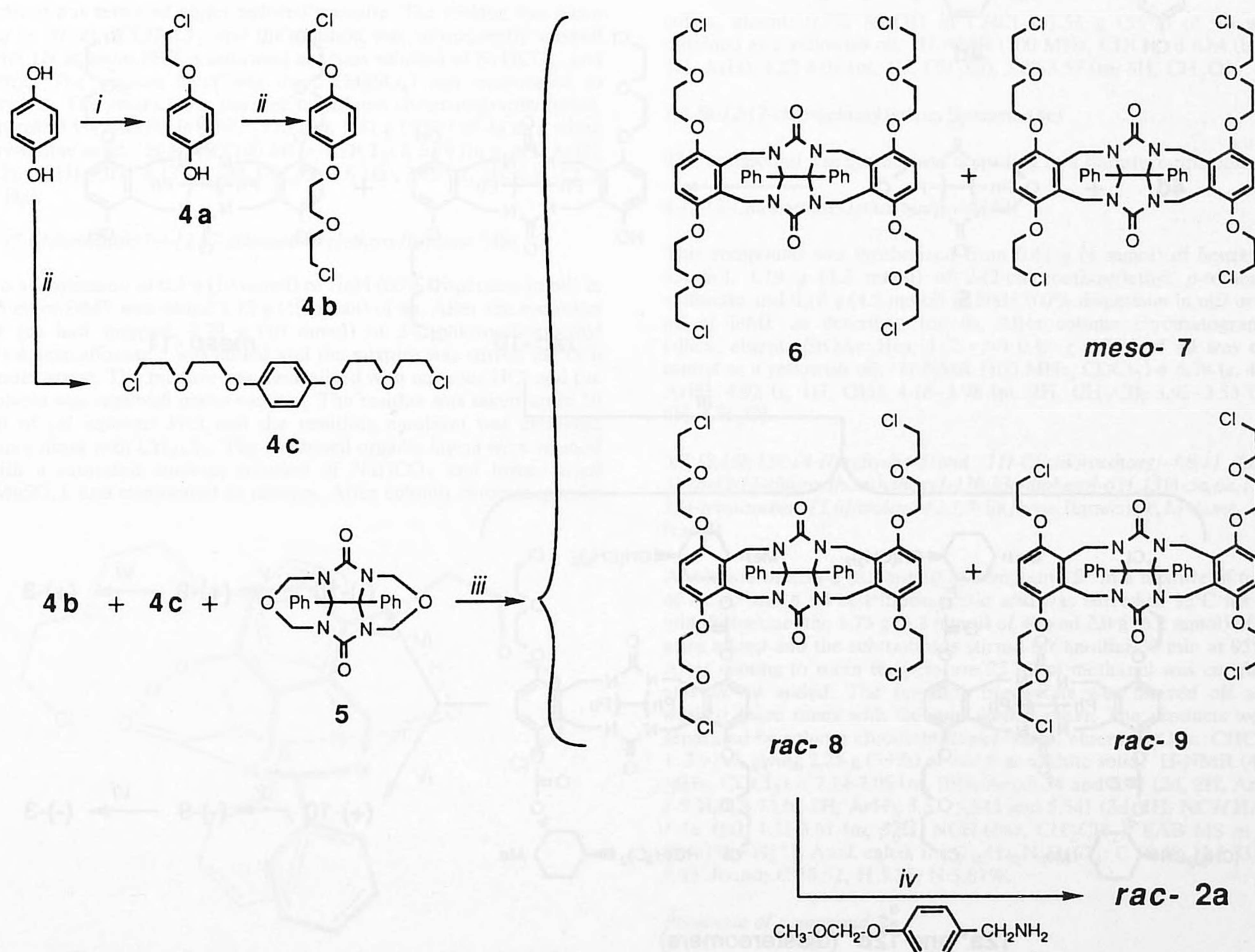
Scheme 1. i) \text{BrCH}_2\text{CH}_2\text{Cl}/\text{K}_2\text{CO}_3 ; ii) \text{TsO}-\text{O}-\text{Cl}/\text{NaH} , DMF; iii) \text{Ac}_2\text{O}/\text{TFA} ; iv) \text{Na}_2\text{CO}_3/\text{NaI} , MeCN.
