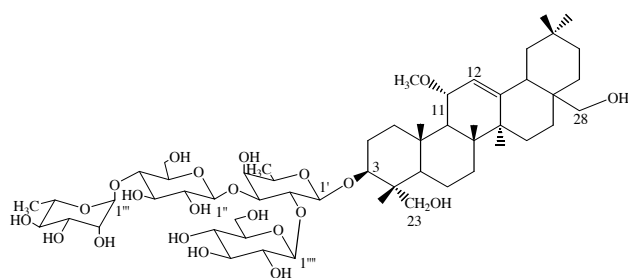
Ilwensisaponin C (6)
