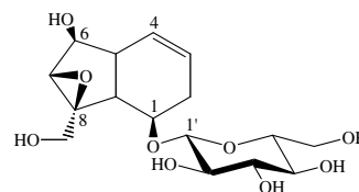
Catalpol (4)
