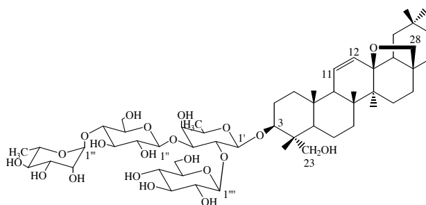
Ilwensisaponin A (5)
