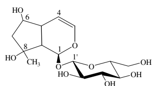
Ajugol (1)
