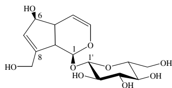
Aucubin (2)
