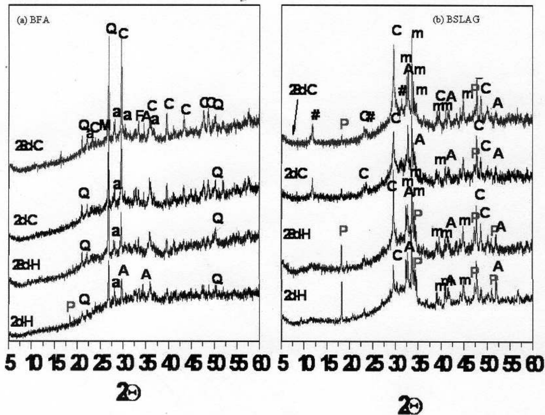
Fig. 4 - Two- and 28-day XRD traces: (a) cement BFA; (b) cement BSLAG / Diffractogramele RX caracteristice pentru paste la 2 zile și la 28 zile: a) ciment BFA; (b) ciment BSLAG.
