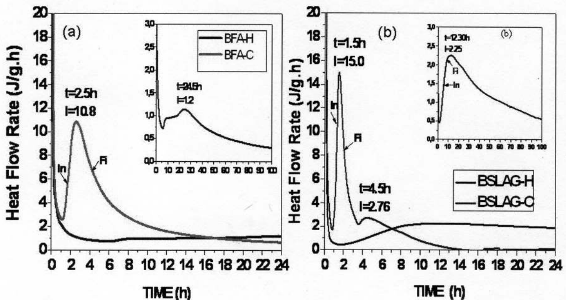
Fig. 1 - Heat flow curves: (a) BFA samples; (b) BSLAG samples; In = initial and Fi =final setting time/ Curbe de încălzire: (a) probe BFA; (b) probe BSLAG ; In = timpul initial și Fi =timpul final de priză.
