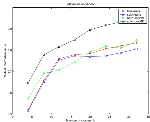
(d) Comparison of MI values for Yahoo20.
