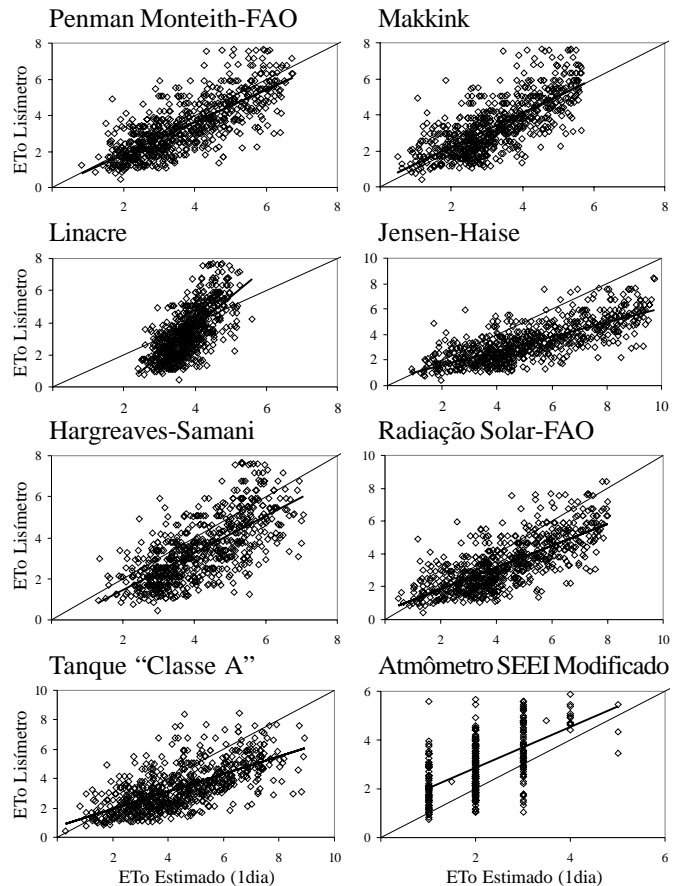
Figura 1. Correlações entre os valores da ETo medidos e estimados, pelos métodos avaliados, em mm dia -1 , no período de 1 dia, na região Norte Fluminense, RJ
