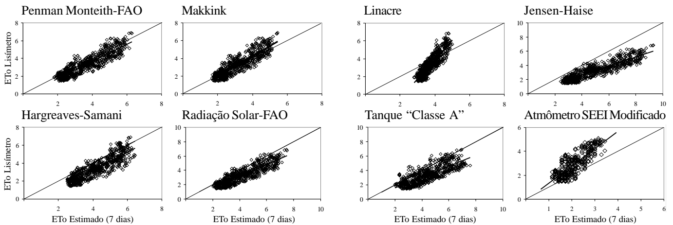
Figura 3. Correlações entre os valores da ETo medidos e estimados pelos métodos avaliados, em mm dia -1 , no período de 7 dias, na região Norte Fluminense, RJ
