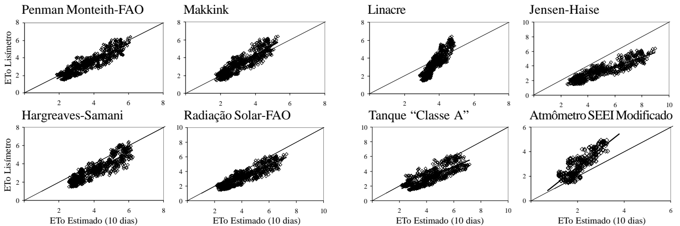
Figura 4. Correlações entre os valores da ETo medidos e estimados pelos métodos avaliados, em mm dia -1 , no período de 10 dias, na região Norte Fluminense, RJ
