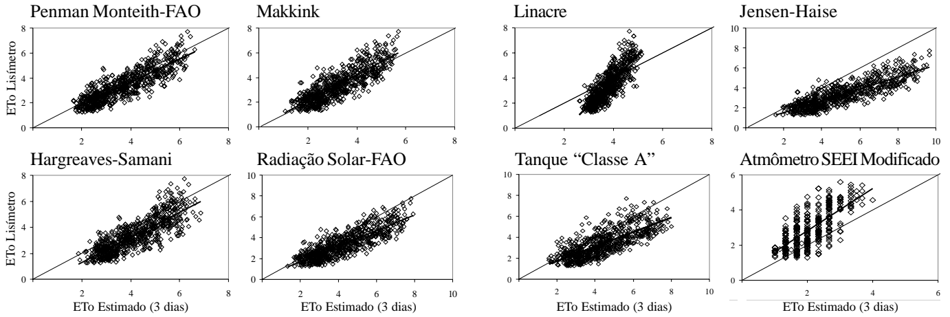
Figura 2. Correlações entre os valores da ETo medidos e estimados pelos métodos avaliados, em mm dia -1 , no período de 3 dias, na região Norte Fluminense, RJ
