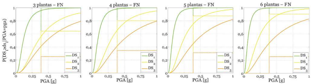
Figura 14. Curvas de fragilidad de los edificios proyectados según PDS-1 para la dirección FN, superpuestas con los daños reales (extraídos de la Figura 4).
