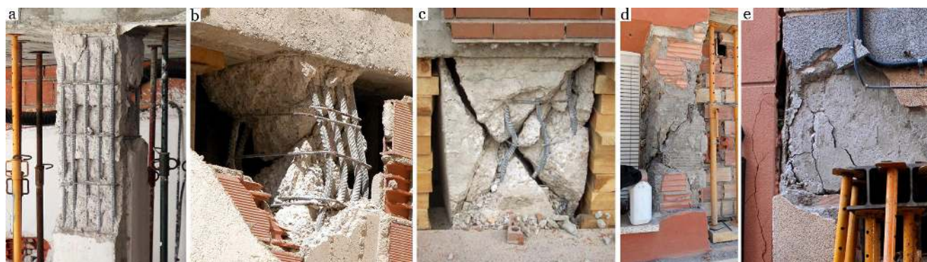
Figura 6. Roturas frágiles (DS4): pilar a cortante por falta de jerarquía (a); pilar a cortante por interacción con la tabiquería (b); pilar corto (c); pilar «cautivo» (d); y nudo a cortante (e).
