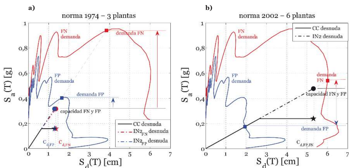
Figura 8. Desempeño de los edificios de 3 plantas calculados según PDS-1 (a) y de 6 plantas según NCSE-02.
