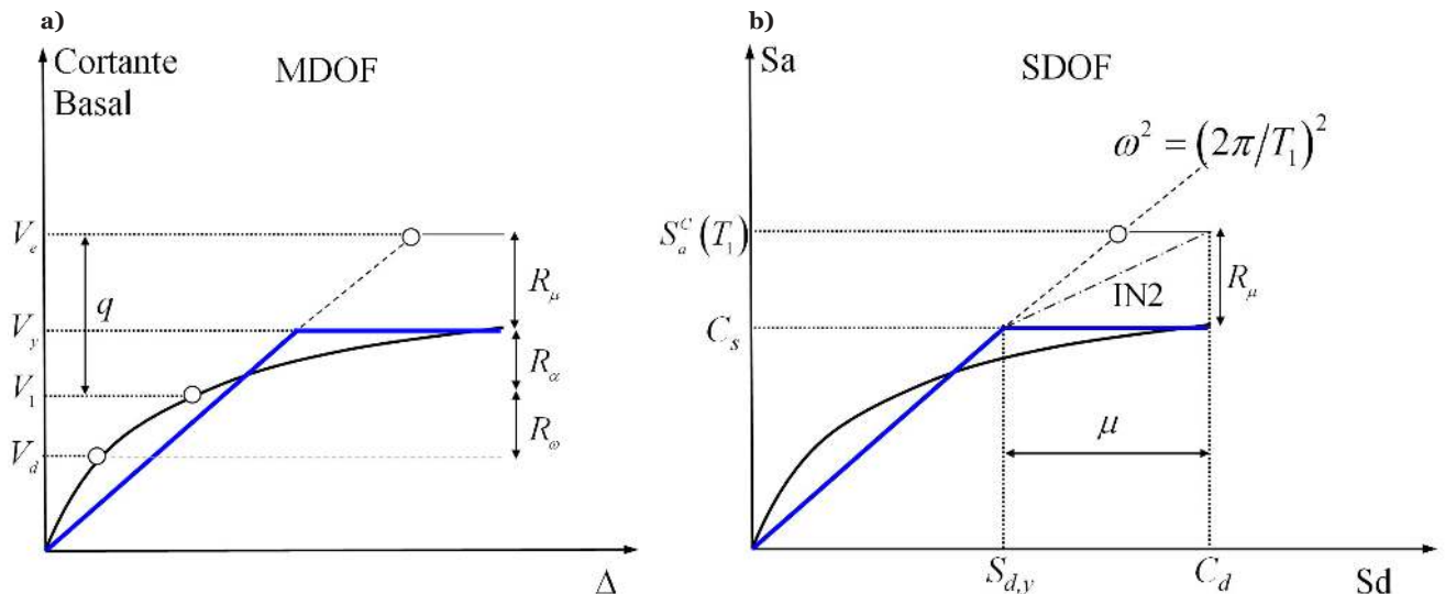
Figura 1. CC idealizada para una estructura desnuda (a) y en formato ADRS con su correspondiente IN2 (b).
