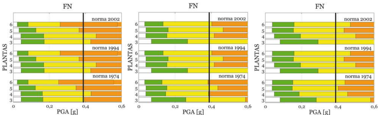
Figura 15. Daño medio esperado en la dirección FN para todas las clases de edificio no uniformemente tabicado, considerando como eficaces los cerramientos y medianeras (a), también la tabiquería insertada en marcos de pórtico (b) y toda la tabiquería (c).
