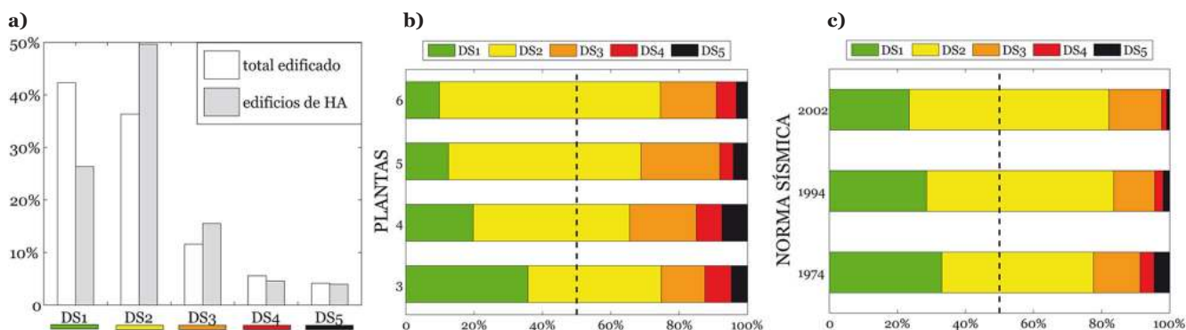
Figura 4. Distribución de frecuencia de DS según EMS-98 para el parque edificado de Lorca (a), para los edificios de HA según el número de plantas (b) y según la norma sísmica aplicada (c) (35).
