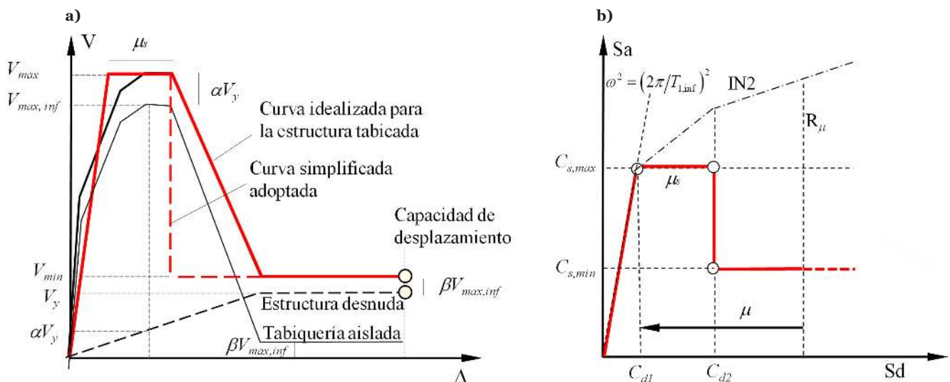
Figura 2. CC aproximada de un edificio de HA tabicado (a), y su representación en formato ADRS (b).
