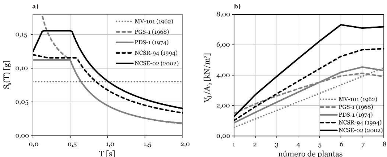
Figura 7. Espectros de proyecto para Lorca (a) y cortante basal normalizado (b).
