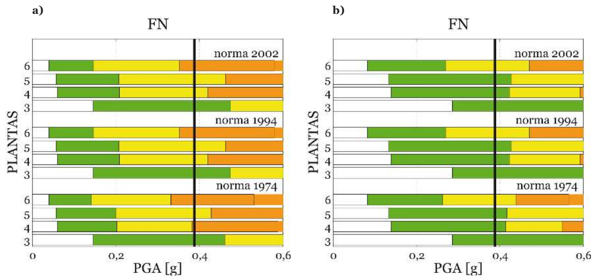
Figura 12. Daño medio esperado para todas las clases de edificio en la dirección FN, para un 1,9% (a) y un 4,2% (b) de tabiquería.
