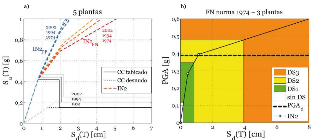
Figura 9. CC e IN2 para edificios tabicados de 5 plantas (a), y daño medio esperado para edificios de 3 plantas según PDS-1 para la dirección FN (b).
