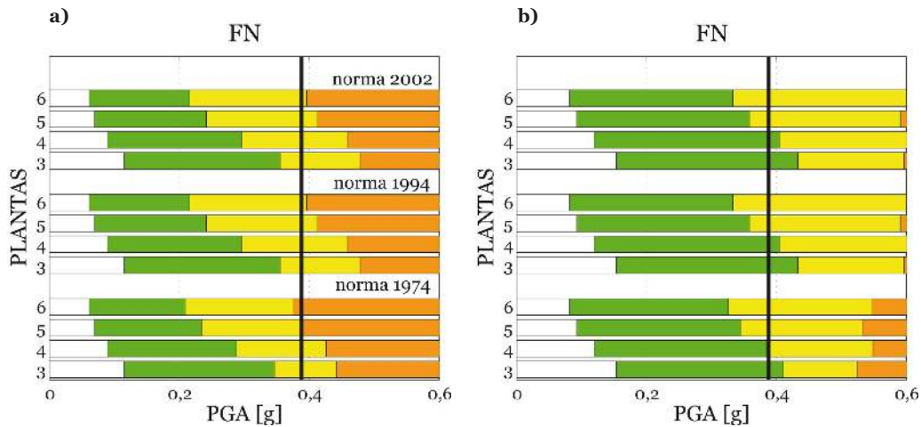
Figura 13. Daño medio esperado para todas las clases de edificio en la dirección FN, para valores de IDR_{DS} en el límite inferior (a) y superior (b).
