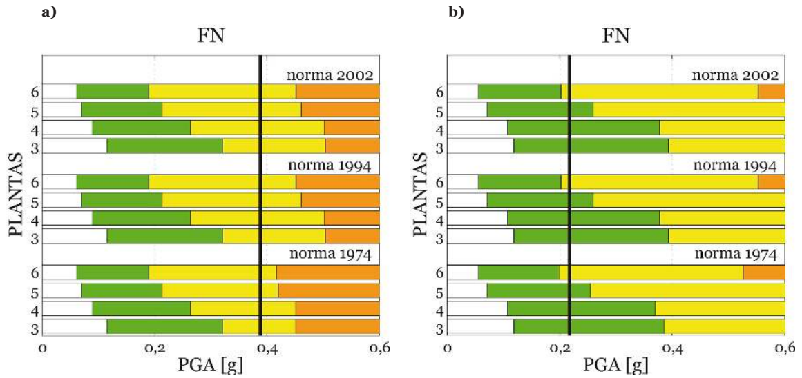
Figura 10. Daño medio esperado para todas las clases de edificio en la dirección FN, para el terremoto principal (a) y para el precursor (b).
