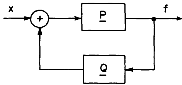
Fig. 23. Feedback system.
