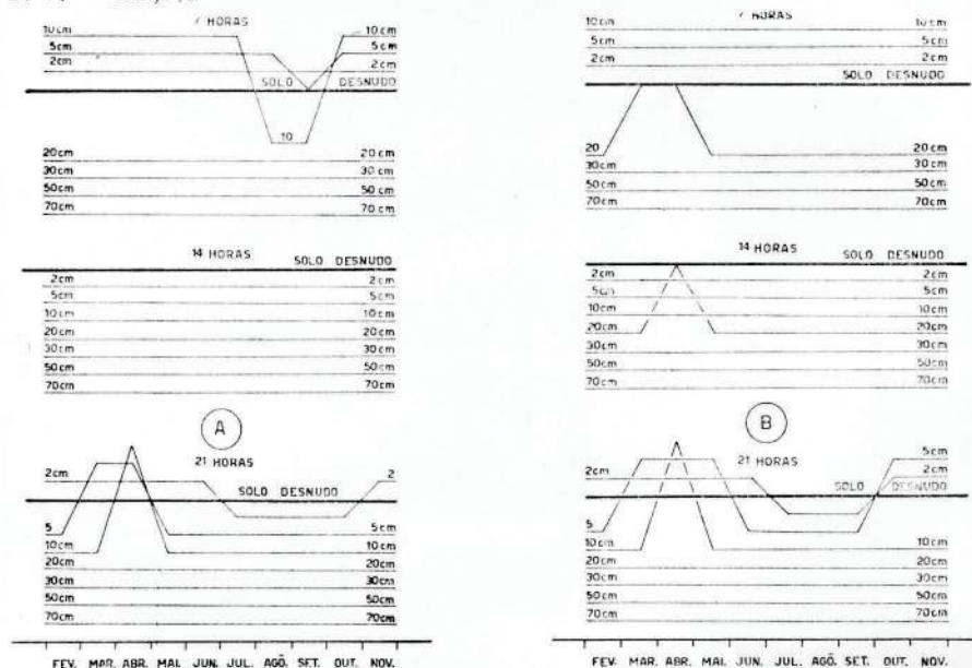
Figura 17 — Representação comparativa das profundidades que apresentam temperaturas superiores ou inferiores às do solo desnudo, durante os meses de fevereiro a novembro de 1955, para as diversas horas de observação. A — solo com cobertura morta. B — solo recoberto com a grama batatais.
