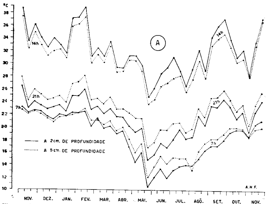
Figura 12 — Temperatura média do solo, em graus Celsius, para diversos decênios do período novembro de 1954 a novembro de 1955, durante horas diversas de observações em solo desnudo. Pósto Meteorológico da Estação Experimental de Ribeirão Preto, São Paulo. A — Temperatura às profundidades de 2 a 5 cm. B — Temperatura às profundidades de 10 a 20 cm.
