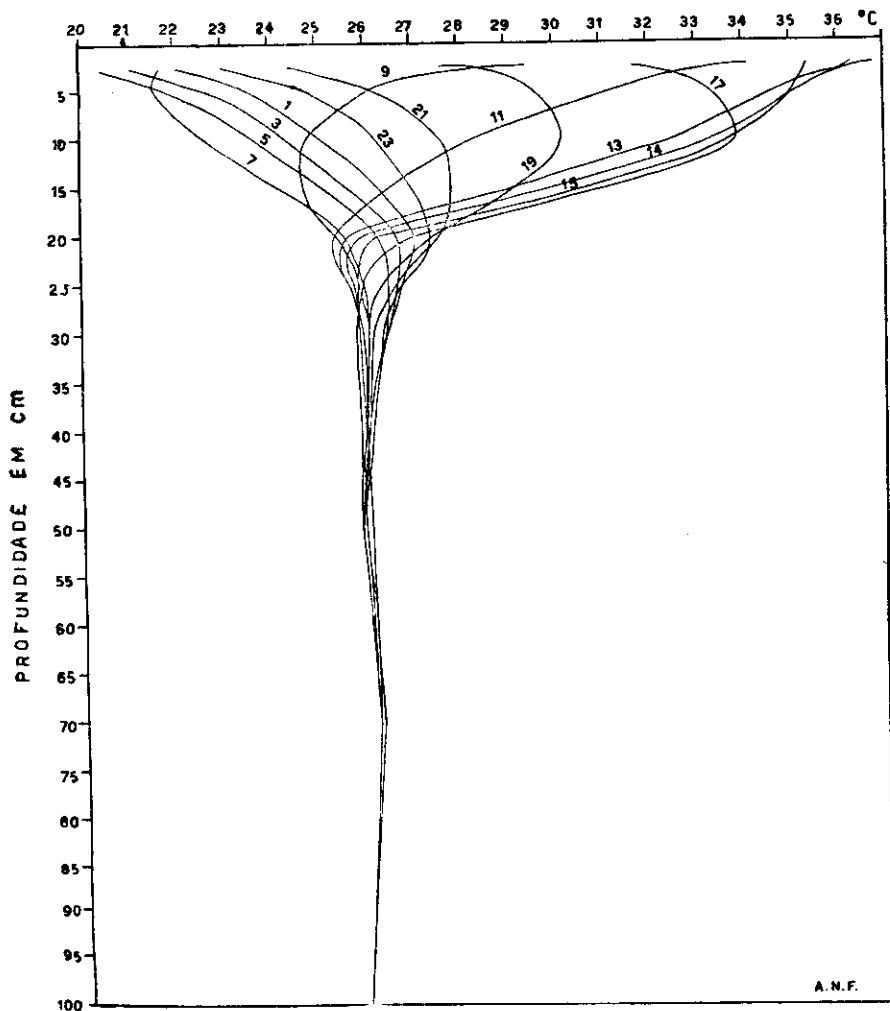
Figura 5 — Tautócronos de temperaturas médias de solo desnudo. Período de 20 a 29 de janeiro de 1955. Pósto Meteoro-Agrário da Estação Experimental de Ribeirão Prêto, São Paulo.
