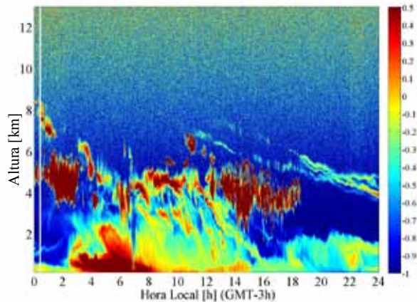
Figura 7. Evolución de la capa límite atmosférica y de las capas de aerosoles para el día 9 de junio de 2011, medido con el sistema lidar en 1064 nm.
