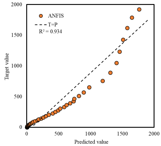
Scen. 2 (Cases, ANFIS)
