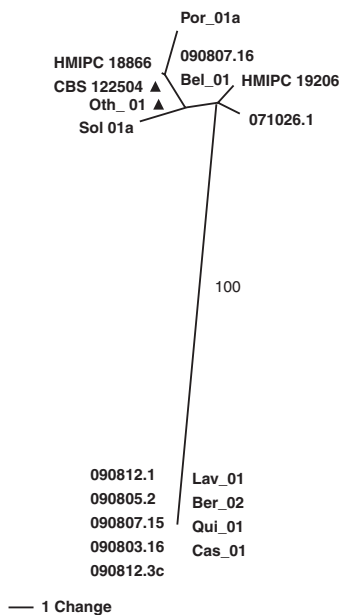
(d) ISSR-PCR
