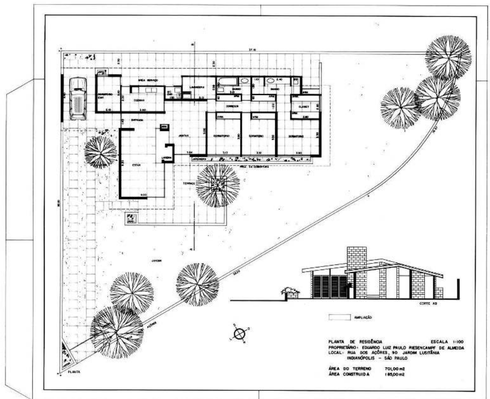
Figura 2. Planta de la primera casa del arquitecto, Residencia calle dos Açores, barrio Jardim Lusitânia, São Paulo, 1958-60 Fuente: Almeida (1958).
