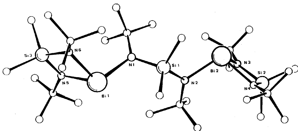
Abb. 3 Zeichnerische Darstellung des Moleküls [\text{Me}_2\text{Si}(\text{N}^t\text{Bu})_2\text{Bi}]_2(\text{N}^t\text{Bu})_2\text{SiMe}_2 ( 6 ) mit einigen Atombezeichnungen.
