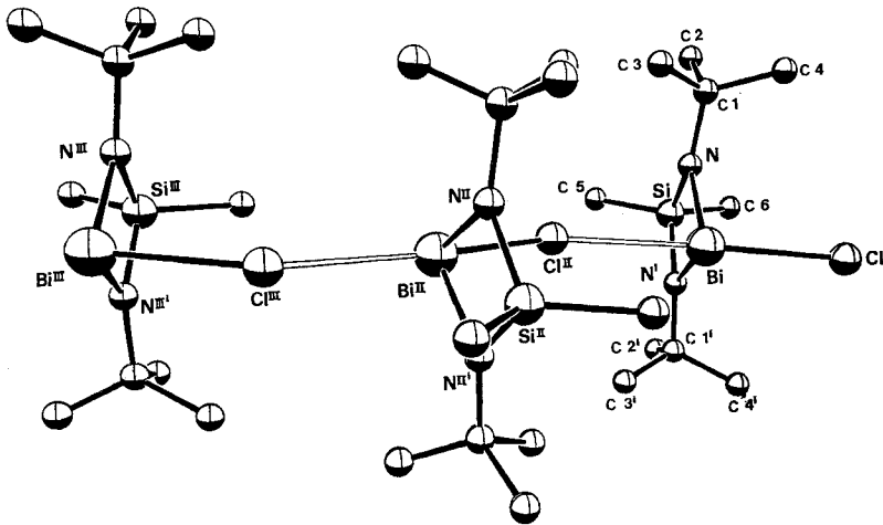
Abb. 2 Ausschnitt aus der Kristallstruktur von \text{Me}_2\text{Si}(\text{N}^t\text{Bu})_2\text{BiCl} (5) mit Atombenennungen. Die mit i bezeichneten Atome gehen aus den unbezeichneten durch die Spiegelebene hervor. Das Molekül II entsteht über eine Gleitoperation, das Molekül III über Translation.
