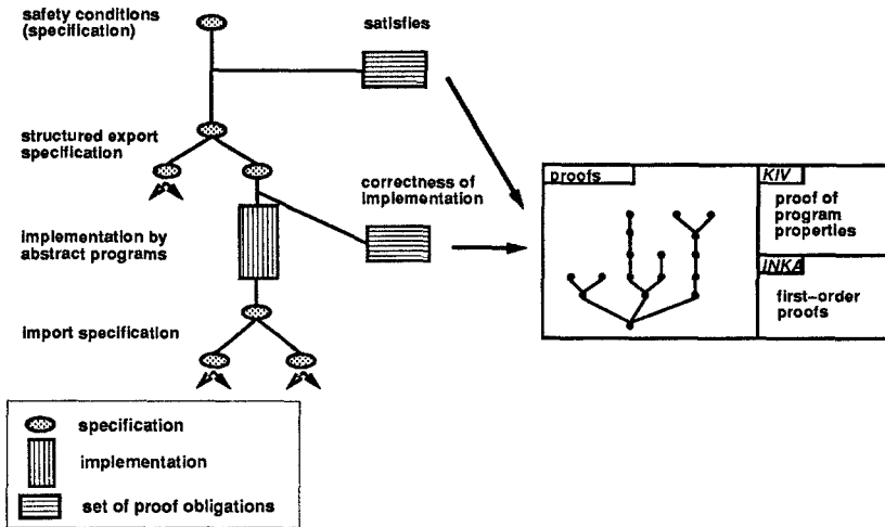
Fig. 1. The VSE Method
