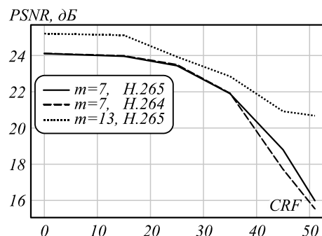
Рис. 12. График зависимости среднего значения PSNR на тестовой выборке от CRF
