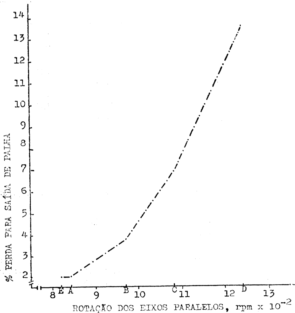
FIGURA 1. Relação entre as rotações dos eixos paralelos e a perda para saída de palha no sistema de debulhamento e limpeza.
