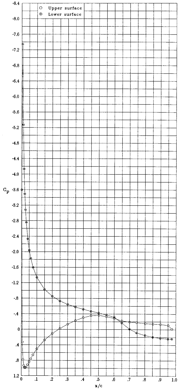
(d) \alpha = -10.15^\circ ; c_l = -0.482 ; c_d = 0.0121 ; c_m = -0.125 .
