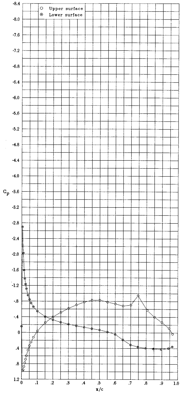
(d) \alpha = -8.11^\circ ; c_l = 0.387 ; c_d = 0.0080 ; c_m = -0.234 .
