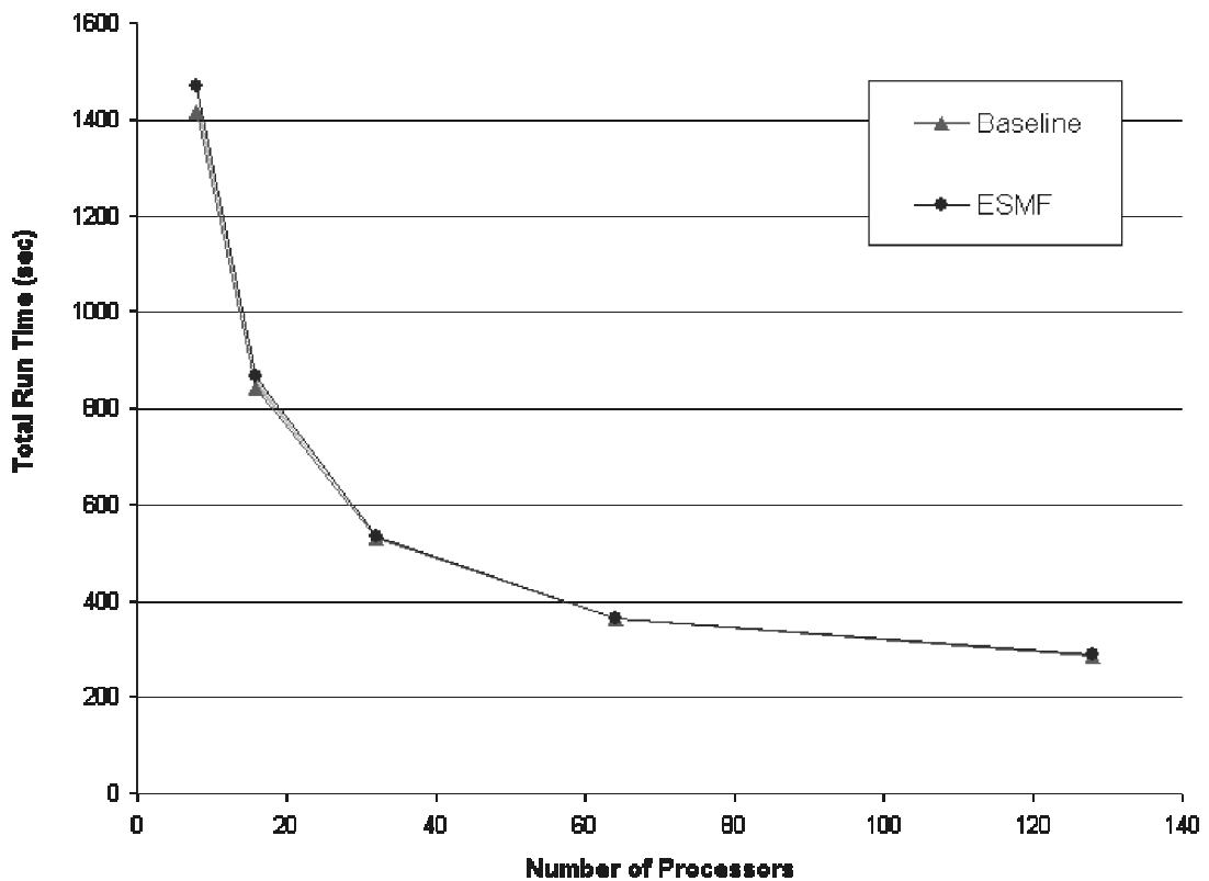
Fig. 3 ESMF overhead in the NCEP SSI.
