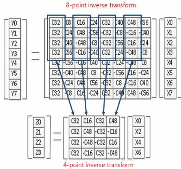
Fig. 4. Relationship between larger size and smaller size blocks in HEVC core transform 그림 4. HEVC 코어 변환에서 상위 크기 블록과 하위 크기 블록 사이의 관계
