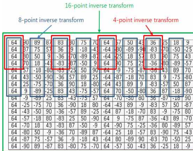
Fig. 5. Coefficients of 16-point HEVC core transform 그림 5. 16-point HEVC 코어 변환의 계수
