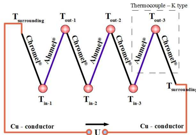
Figure 6. Connection of K type thermocouples Slika 6. Priključak termoparova tipa K
