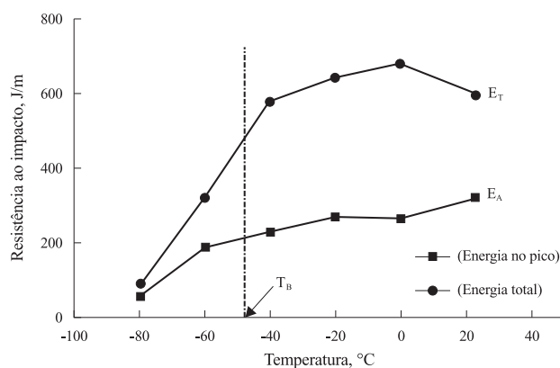
Figura 5. Resistência ao impacto do ABS ilustrando variação de energia no pico e na fratura em função da temperatura. Izod – ASTM D256.
