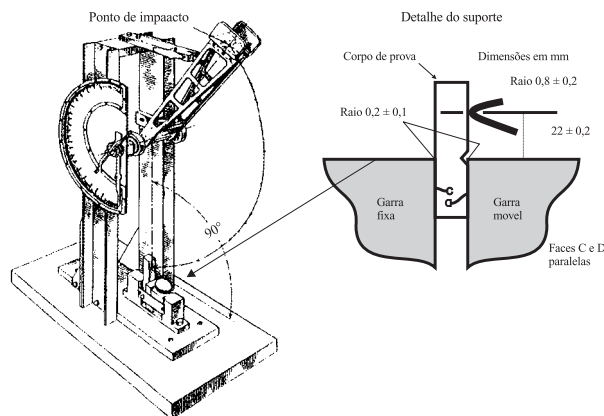
Figura 2. Representação esquemática do ensaio IZOD. Ref. ASTM D256
