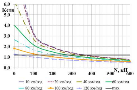
Рис. 3. Коефіцієнт запасу стійкості від витискання порожнього піввагона з урахуванням і без урахування сил тертя в контакті гребеня колеса й рейки відповідно:
