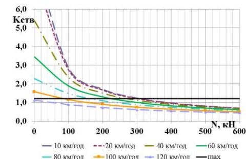
Рис. 3. Коефіцієнт запасу стійкості від витискання порожнього піввагона з урахуванням і без урахування сил тертя в контакті гребеня колеса й рейки відповідно:
