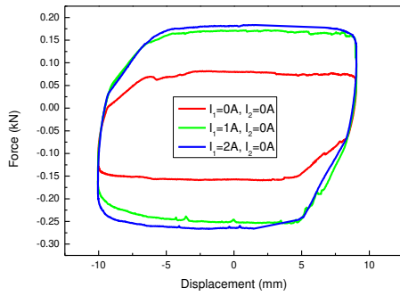
Fig.10. Variable damping
