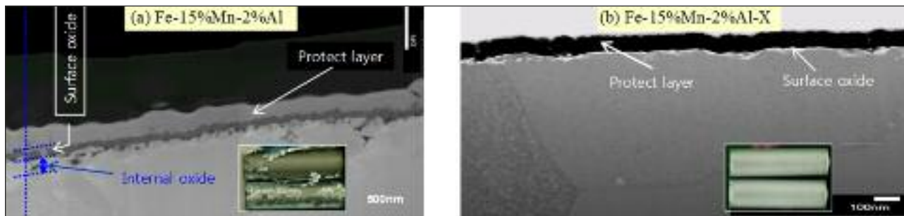
FIG. 4 Effects of some alloying elements on surface oxide layer and coating adhesion. Effetti di alcuni elementi alliganti sullo strato di ossido superficiale e sull'adesione del rivestimento.
