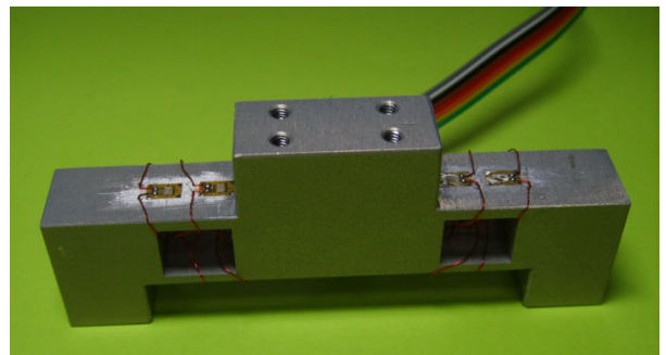
그림 7. 제작된 2축 힘/모멘트센서의 사진. Fig. 7. Photograph of manufactured two-axis force/moment sensor.
