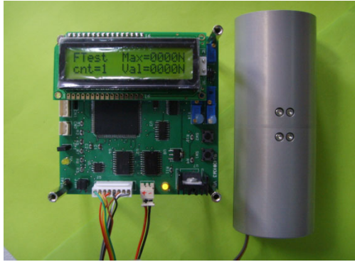
그림 11. 제작된 원통형 손가락 힘측정장치의 사진. Fig. 11. Photograph of manufactured cylindrical-type finger force measuring system.
