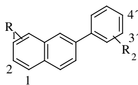
I.B, I.7, I.8, I.9, I.11
