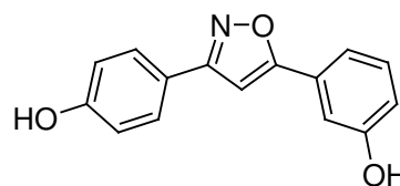
IC_{50} (HSD2) = 270 nM
