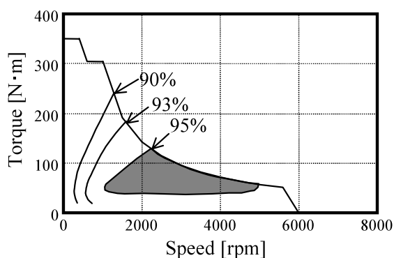
Fig. 18. 2000 Prius motor loss map
