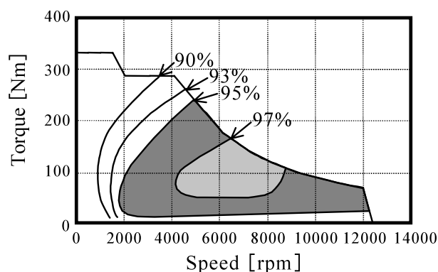
Fig. 19. 2005 SUV motor loss map
