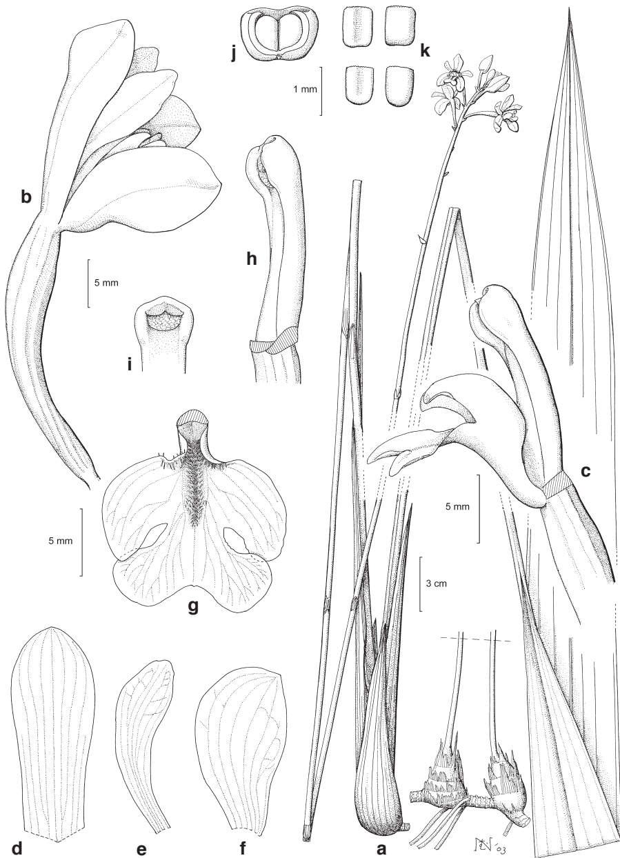
Fig. 1. Devogelia intonsa Schuit. a. Habit; b. flower; c. lip and column; d. median sepal; e. petal; f. lateral sepal; g. lip; h. column; i. column apex in ventral view; j. anther; k. pollinia (all: De Vogel 4175).
