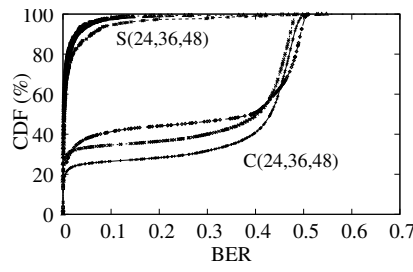
Fig. 5. CDF of Bit-Error Rate (BER)
