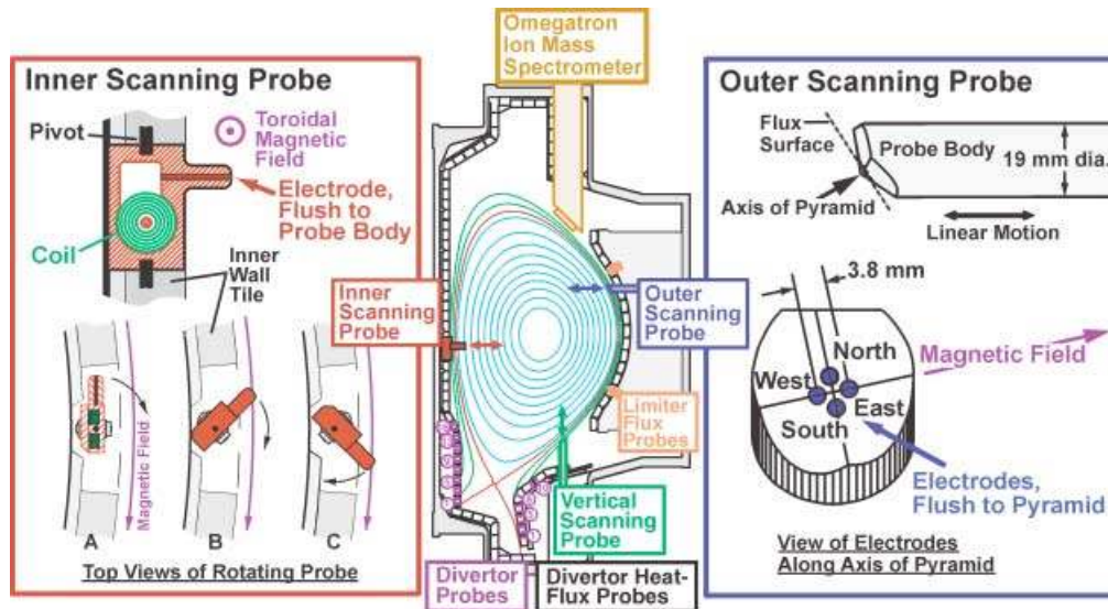
Fig. 25. Probe diagnostics on C-Mod.
