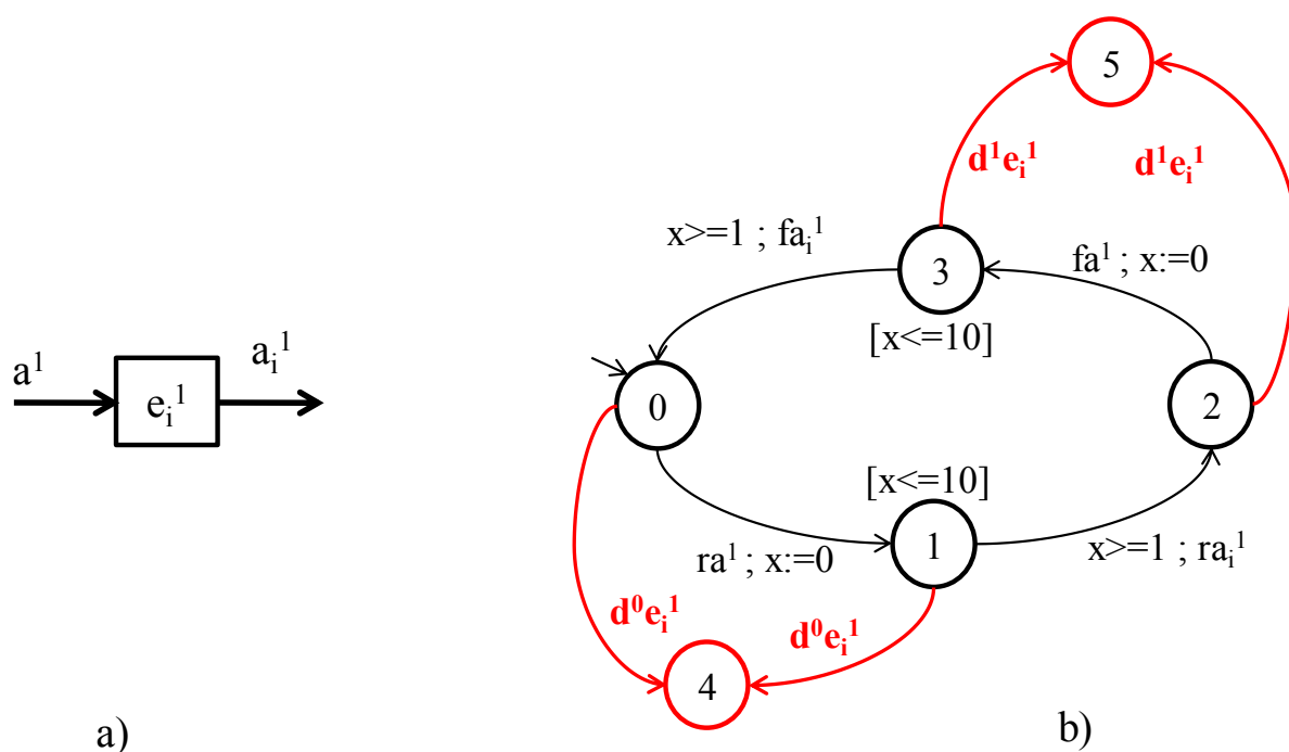
Figure C-2 : Modèle Comportemental du port d'entrée e_i^1
