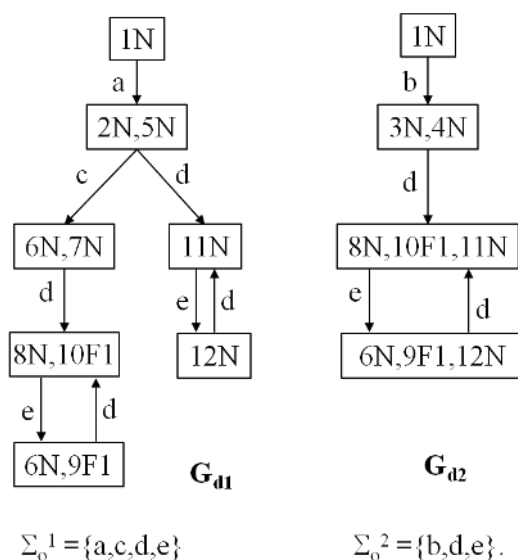
Figure III-9 – Diagnosticheurs des deux sites surveillant le système de la Figure III-8
