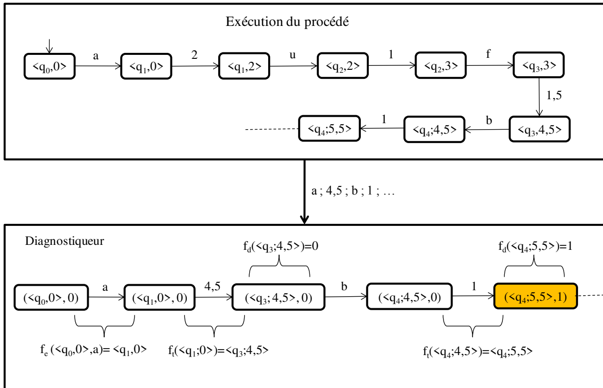
Figure IV-9 – Diagnostiqueur par estimation d'état
