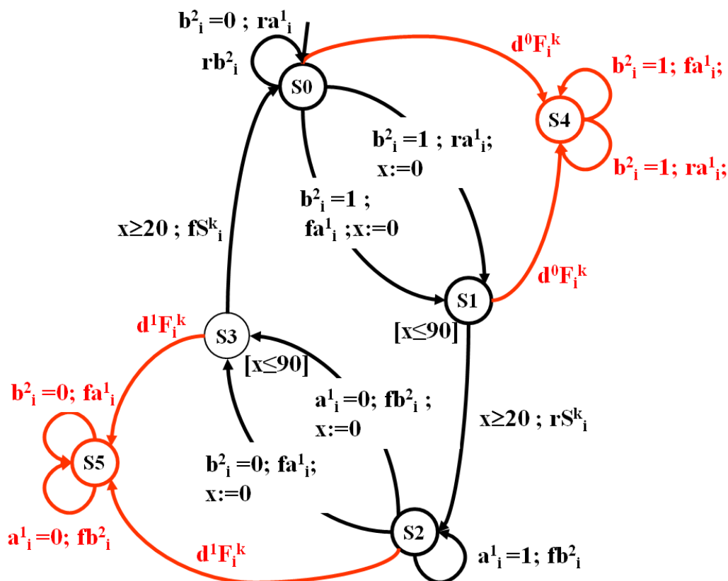
Figure V-20 – Modèle de comportement complet d'un composant logique à deux entrées
