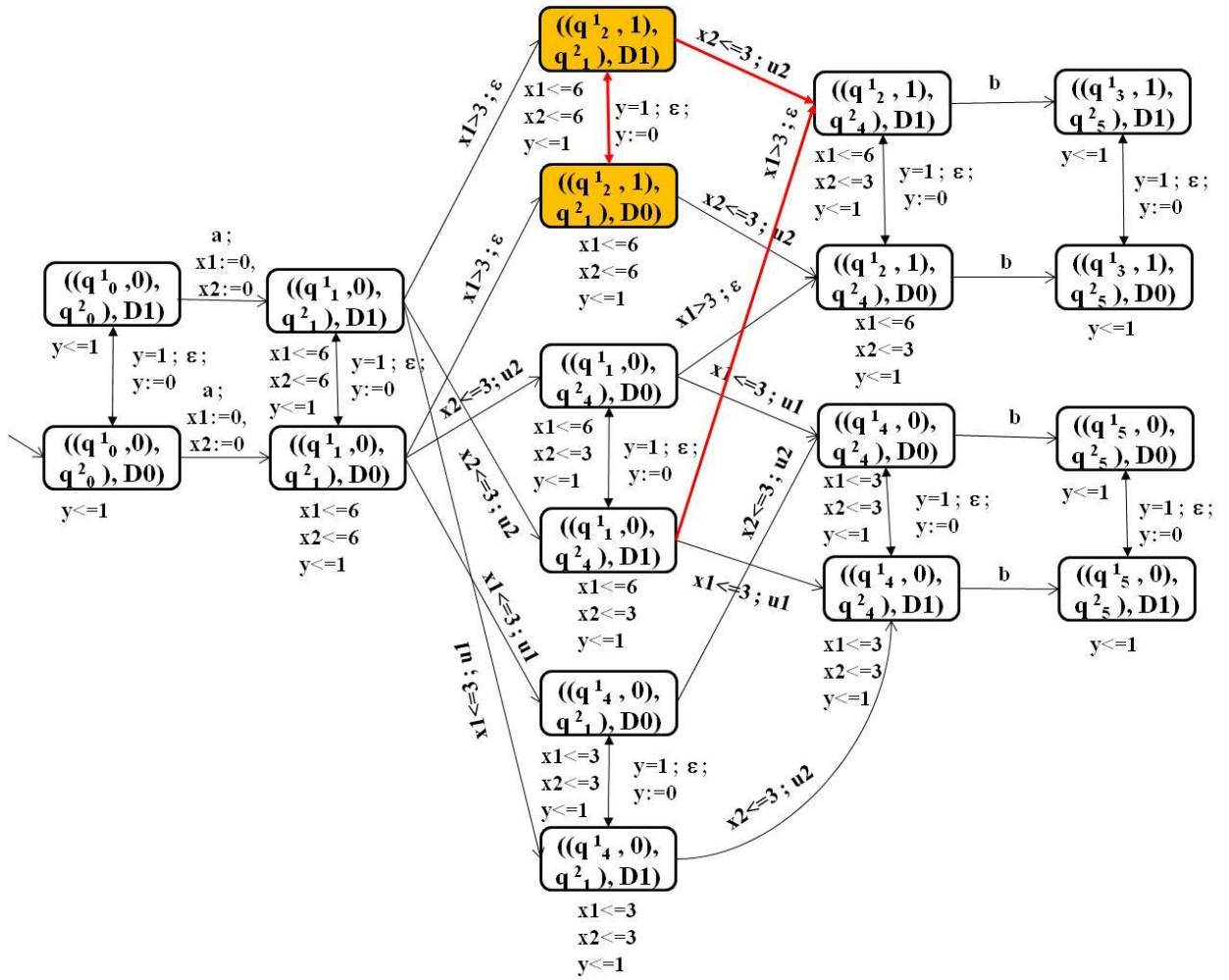
Figure IV-8 – Automate D obtenu à partir de l'exemple de Figure IV-1
