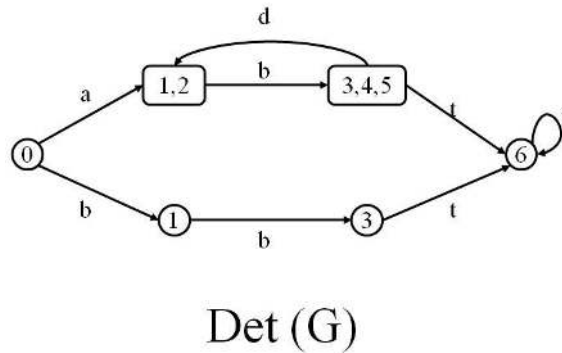
Figure II-5 – Automate déterminisé de l'exemple de la Figure II-3
