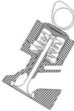
b) Tappet
