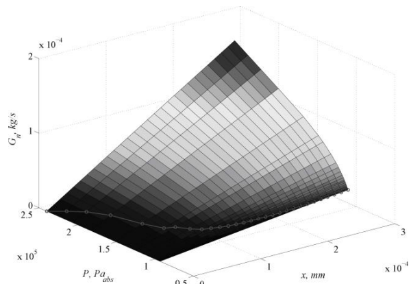
Fig. 13. Variación total del flujo de masa G_n . Fuente: Autores
