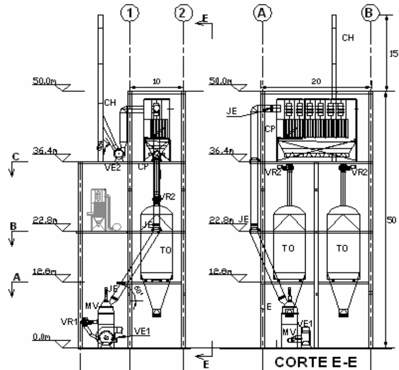
Figura 2. Planta de Molienda Desarrollada
