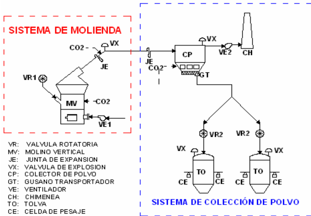
Figura 1. Flujograma de la Planta de Molienda.
