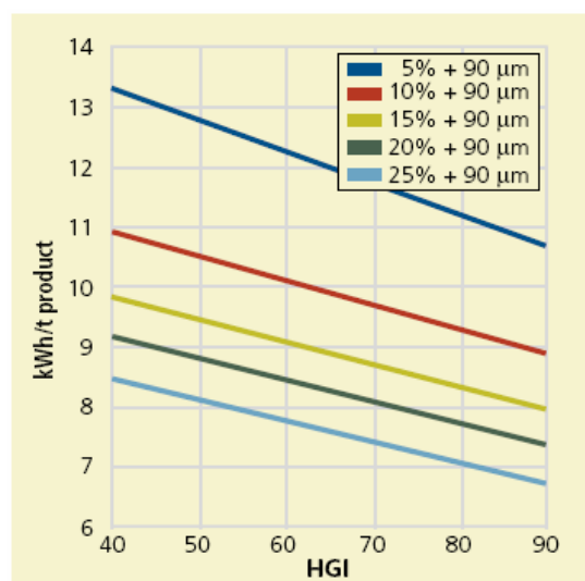
Figura 3. Potencia del Molino según Índice de Molturabilidad HGI [1]
