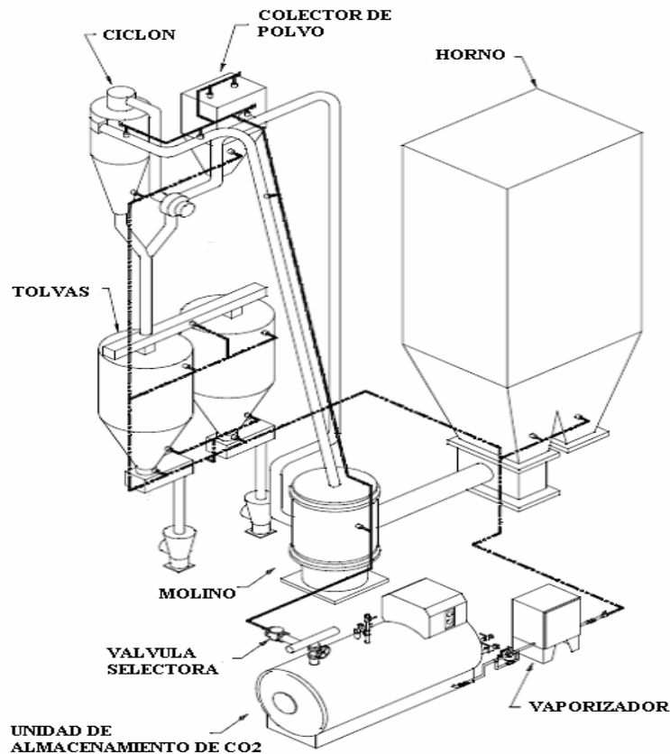
Figura 4. Esquema del Sistema de Inertización por CO 2 para un Sistema de Molienda de Carbón Mineral
