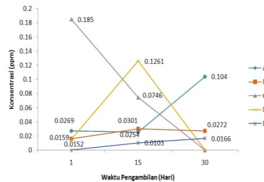
Gambar 1. Kandungan logam merkuri dalam sedimen pada 5 titik dengan waktu pengambilan 1, 15, dan 30 hari.
