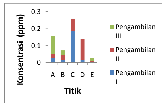
Gambar 2. Konsentrasi Hg total pada 5 titik dengan waktu pengambilan I (hari ke 1), II (hari ke 15), dan III (hari ke 30)
