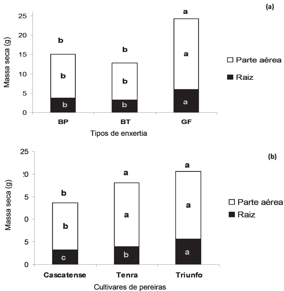
FIGURA 1- Produção de matéria seca da raiz, da parte aérea e total em função dos métodos de enxertia em mudas de pereira (BP: borbulhia em placa; BT: borbulhia em ‘T’ invertido; GF: garfagem de fenda cheia) – (A) e cultivares de pereira ‘Cascatense’, ‘Tenra’ e ‘Triunfo’ (B). Para cada parte e total, médias seguidas pela mesma letra não diferem entre si, a 5%, pelo teste de Tukey.
