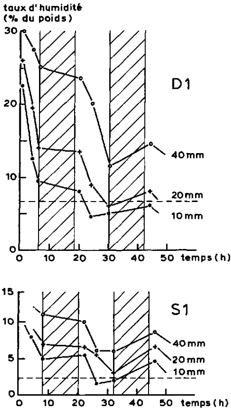
Fig. I.3.7. Taux d'humidité dans la couche superficielle du sol (épaisseur 1,5 cm) - sol limon sableux (sable S1), après des pluies artificielles de 10, 20 et 40 mm, à 10 h du matin (14, 15, 16 Juillet 1980). (Taux d'humidité du sol avant la pluie 1%.) - sol argileux (argile D1) après des pluies artificielles de 10, 20 et 40 mm à 12 h (14, 15, 16 Juillet 1980). (Taux d'humidité du sol avant la pluie 2%.) (---- point de flétrissement des plantules des graminées dominantes.) Remarque: les bandes hachurées correspondent aux heures de la nuit.
