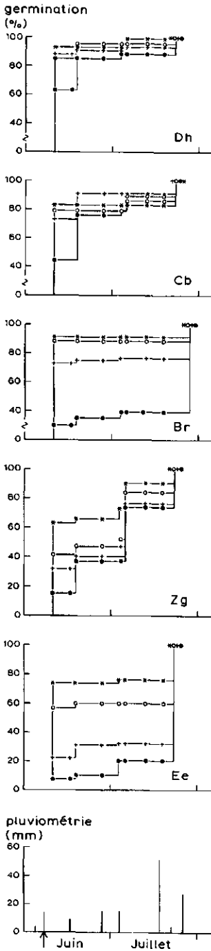
Fig. II.1.12. Courbes de germination des espèces dominantes suivant la pluviométrie. Station sable S1, 1980. La date des pluies artificielles de 0 mm (●), 10 mm (+), 20 mm (○) et 40 mm (*) a été indiquée par une flèche. Diheteropogon hagerupii (Dh), Cenchrus biflorus (Cb), Borreria radiata (Br); Zornia glochidiata (Zg); Elionurus elegans (Ee). NB. Les nombres des germinations cumulés sont indiqués en figure II.1.11.
