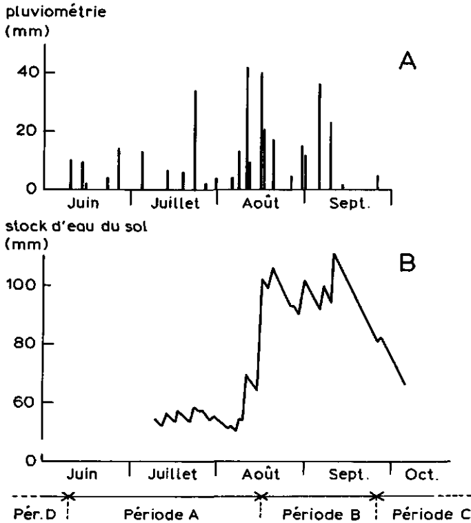
Fig. I.3.5 Pluviométrie, stock de l'eau du sol et subdivision de l'année en périodes suivant l'activité des plantes, les précipitations et l'eau du sol. Station sable S2, 1977. A = pluviométrie journalière B = stock de l'eau du sol (selon Penning de Vries et Djitéye, 1982, p. 160).
