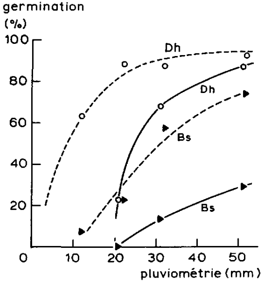
Fig. II.1.15. Le taux de germination en rapport avec la hauteur de la première pluie pour Dheteropogon hagerupii (Dh) et Borreria stachydea (Bs) sur S1 (----) et D1 (—).
