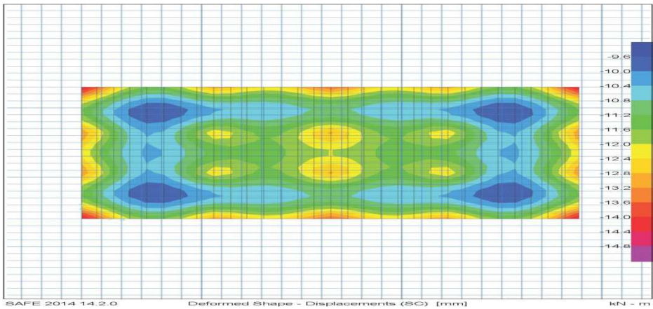
Fig. 7. Raft deformations ( K_s=15000 kN/m 3 ).
