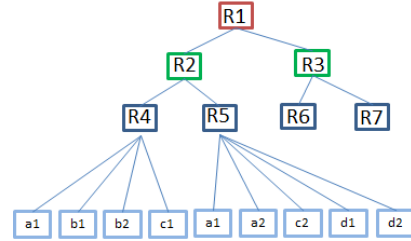
Fig. 2: R-tree
